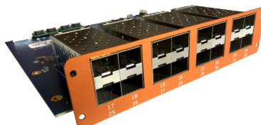
BTF1-41-SFP16 SFP+ 拡張カード
