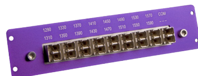
BTF1-41-MUX08/16 CWDM拡張カード
